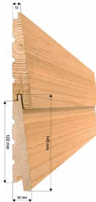
Coffrage incliné rainure+langue (côté visible rugueux ou raboté) (Profil N°3)
